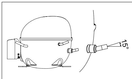
图2 吸气管角度为 15^{\circ}
