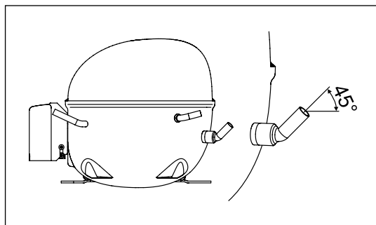
图1 吸气管角度为 45^{\circ}
